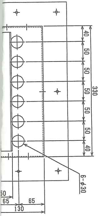
塞ぎ板製作図
