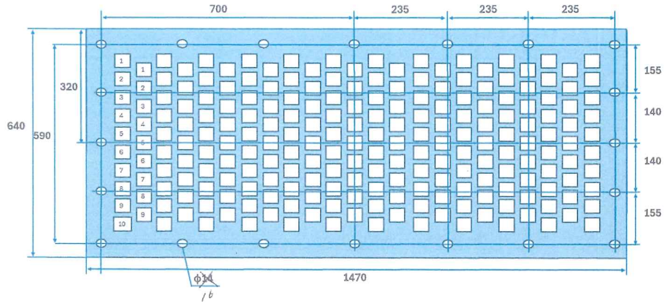
拡大図
